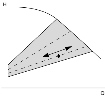
Рис. 30 Новая нижняя кривая пропорционального давления
