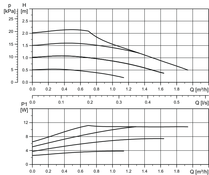
Эксплуатационная характеристика
