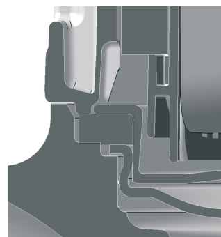
Рис. 44 Чертеж в разрезе с изображением принципа закупоривания уплотнения
