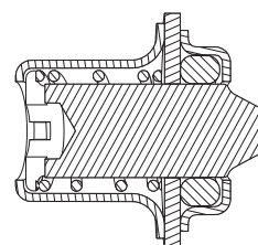
Рис. 37 Вид разблокирующего устройства в разрезе
