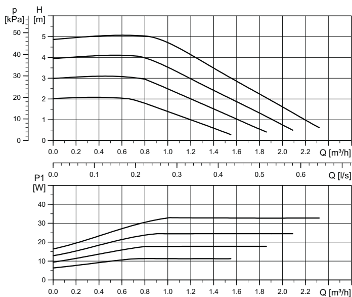
Эксплуатационная характеристика
