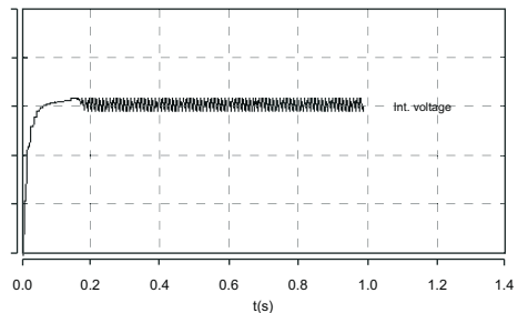
Рис. 56 Пример: Насос UPM3 с внутренним пусковым реле
