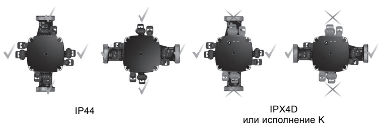
Расположение блока управления
