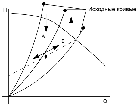
Рис. 29 Рабочая точка на выбранной кривой пропорционального давления.
