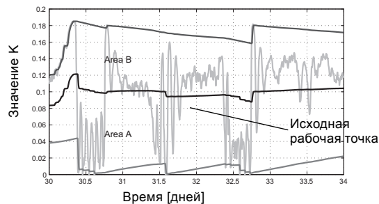
Рис. 28 K_{sys} -значения, зарегистрированные для анализатора системы
