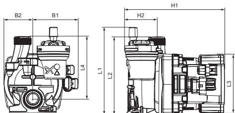
Размеры
