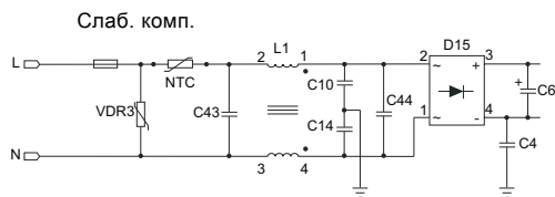
Рис. 54 NTC
