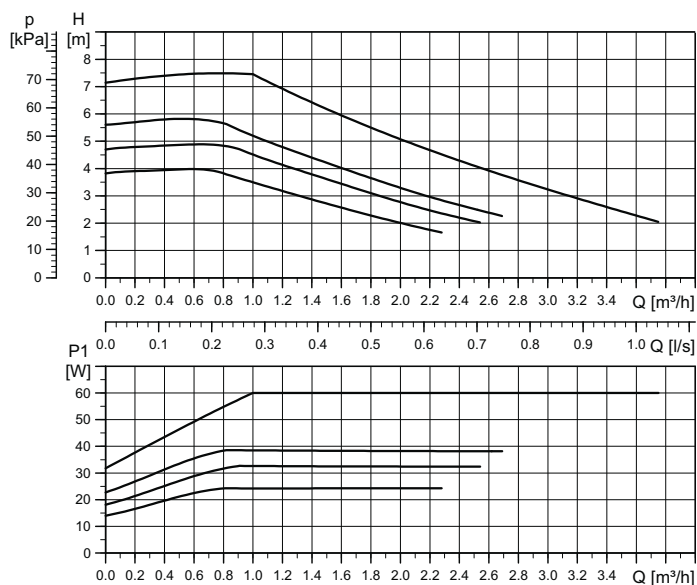
Эксплуатационная характеристика
