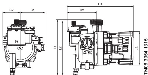
Размеры
