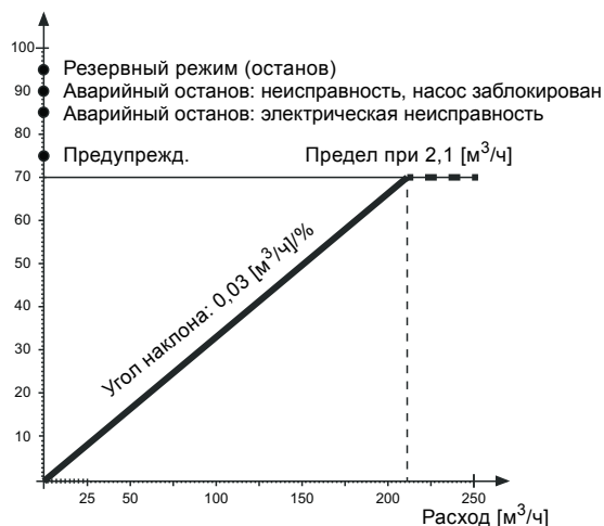
Рис. 16 ШИМ-сигнал обратной связи - определение расхода
